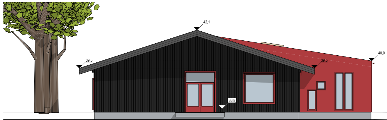
Fasade Øst Nybygg
